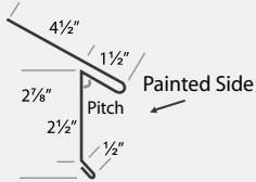
DRIP EDGE
