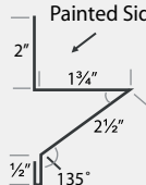
HR BASEGUARD
